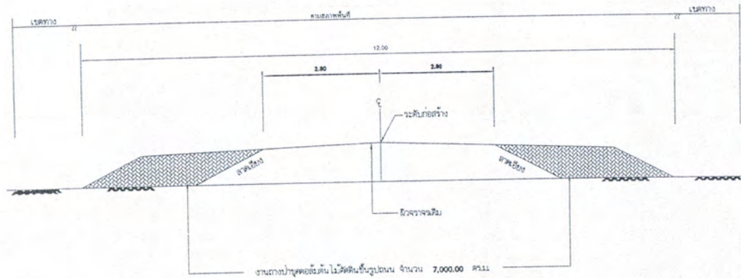
รูปตัดตามขวางแสดงการตัดดินขึ้นรูปได้ดิน(ก่อนดำเนินการ) มาตราส่วน 1 : 50
