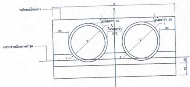
รูปสิ่งปลูกสร้างแบบหน้าตัดคู่ 1:25
