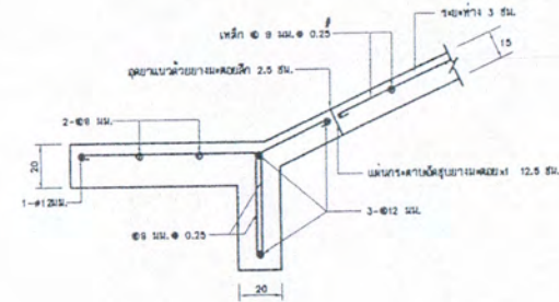
รูปสิ่งปลูกสร้างแบบหน้าตัดเดี่ยว 1:25
