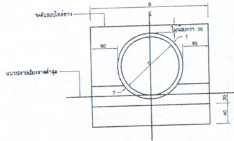
รูปสิ่งปลูกสร้างแบบหน้าตัดเดี่ยว 1:25
