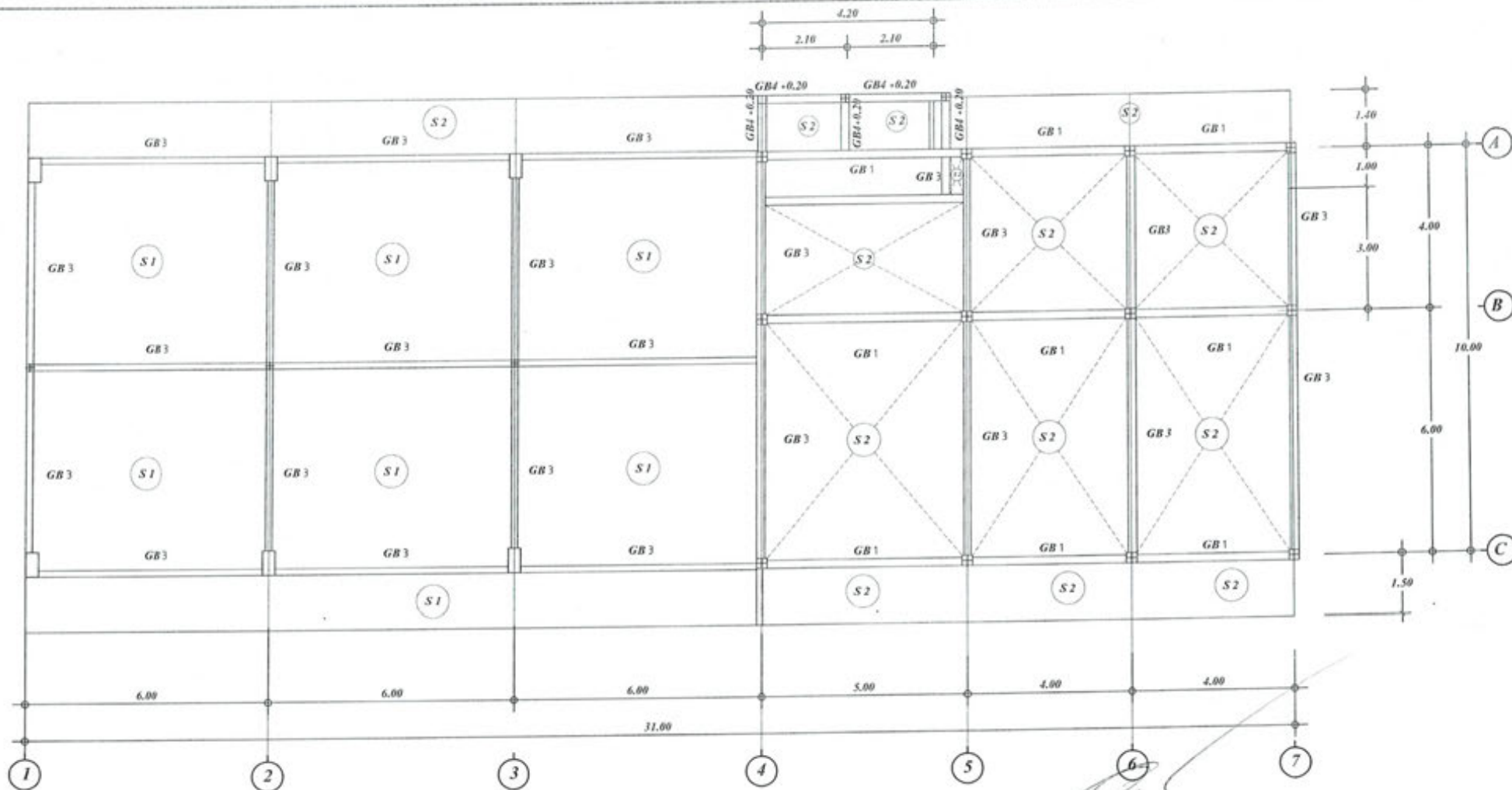
แปลนคานาคอดิน เสา พื้น มาตราส่วน 1 : 100
