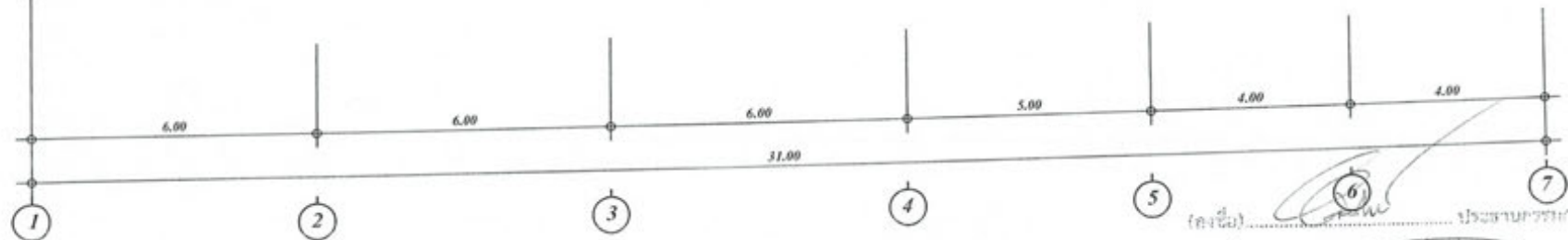
แปลนไฟฟ้าชั้นบน มาตราส่วน 1 : 100
