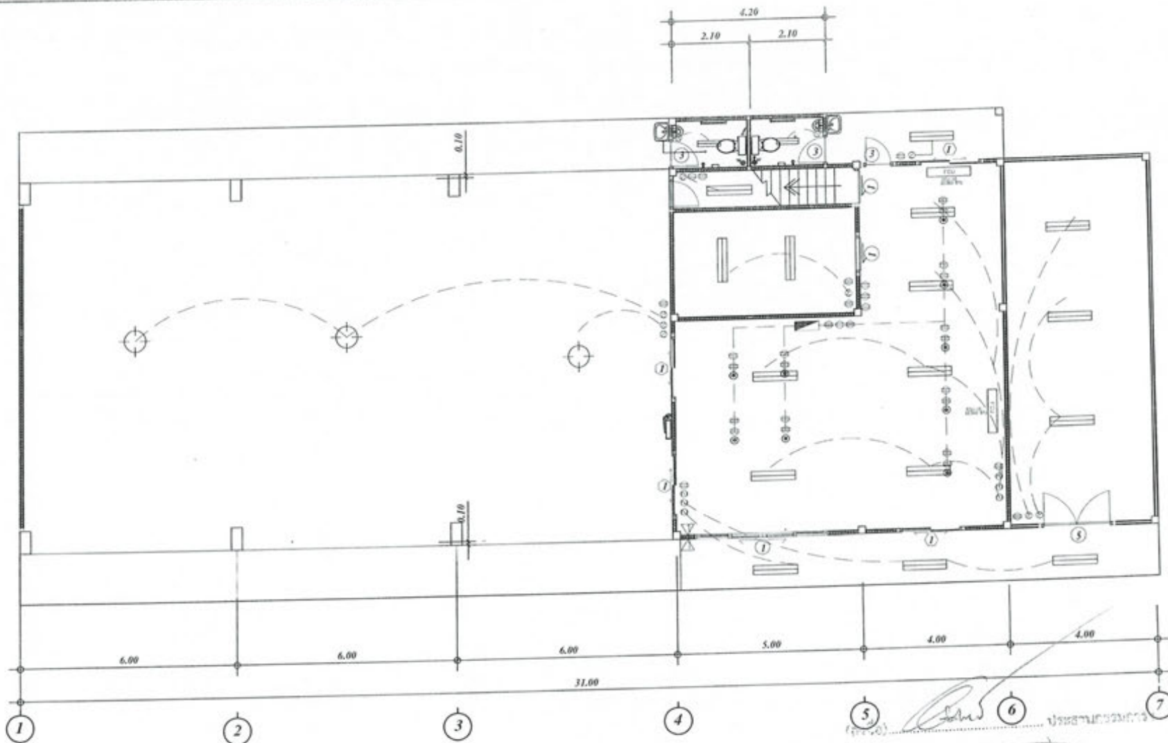
แปลนไฟฟ้าชั้นล่าง มาตราส่วน 1 : 100
