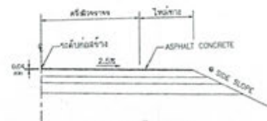
แบบขยายผิวจราจร
