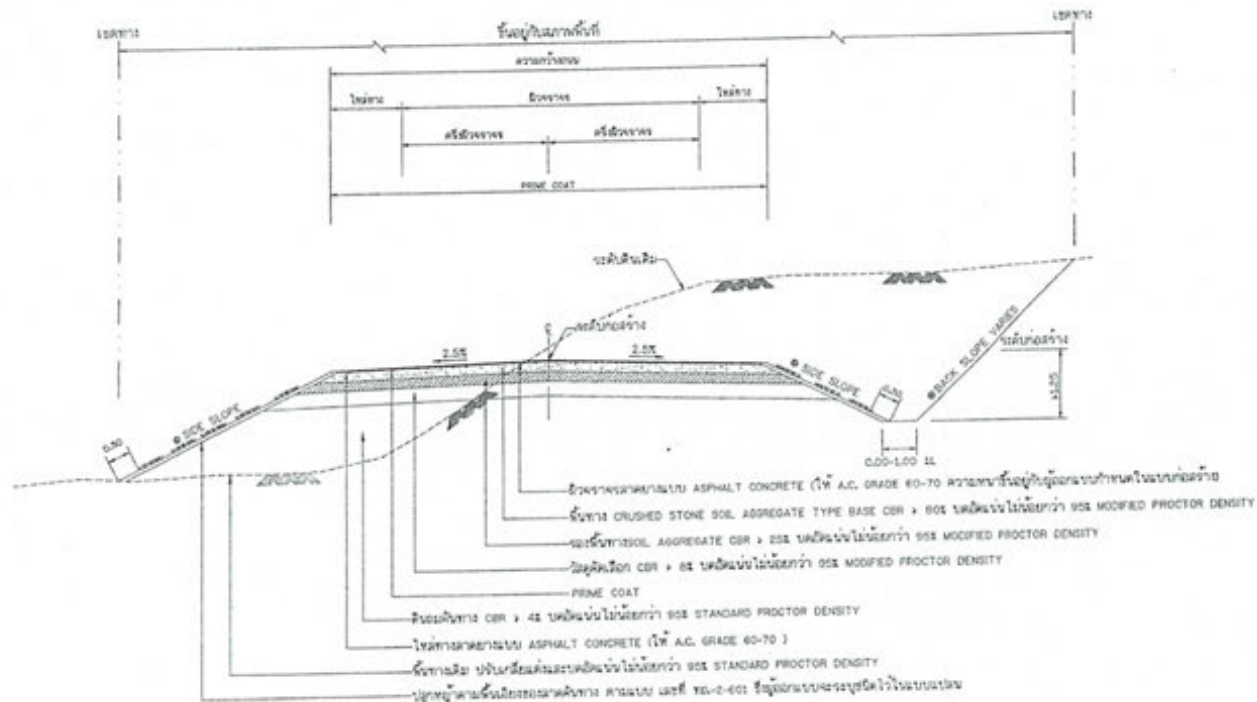
รูปตัดแสดงโครงสร้างถนนดินดิบ ดินถมและคลุมทับผิววัสดุ
