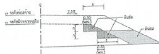
รูปตัดแสดงโครงสร้างลาดชันทางบนถนนเดิม
